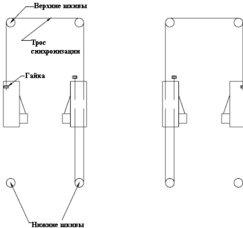
Рис. 2.1 - Установка тросов
