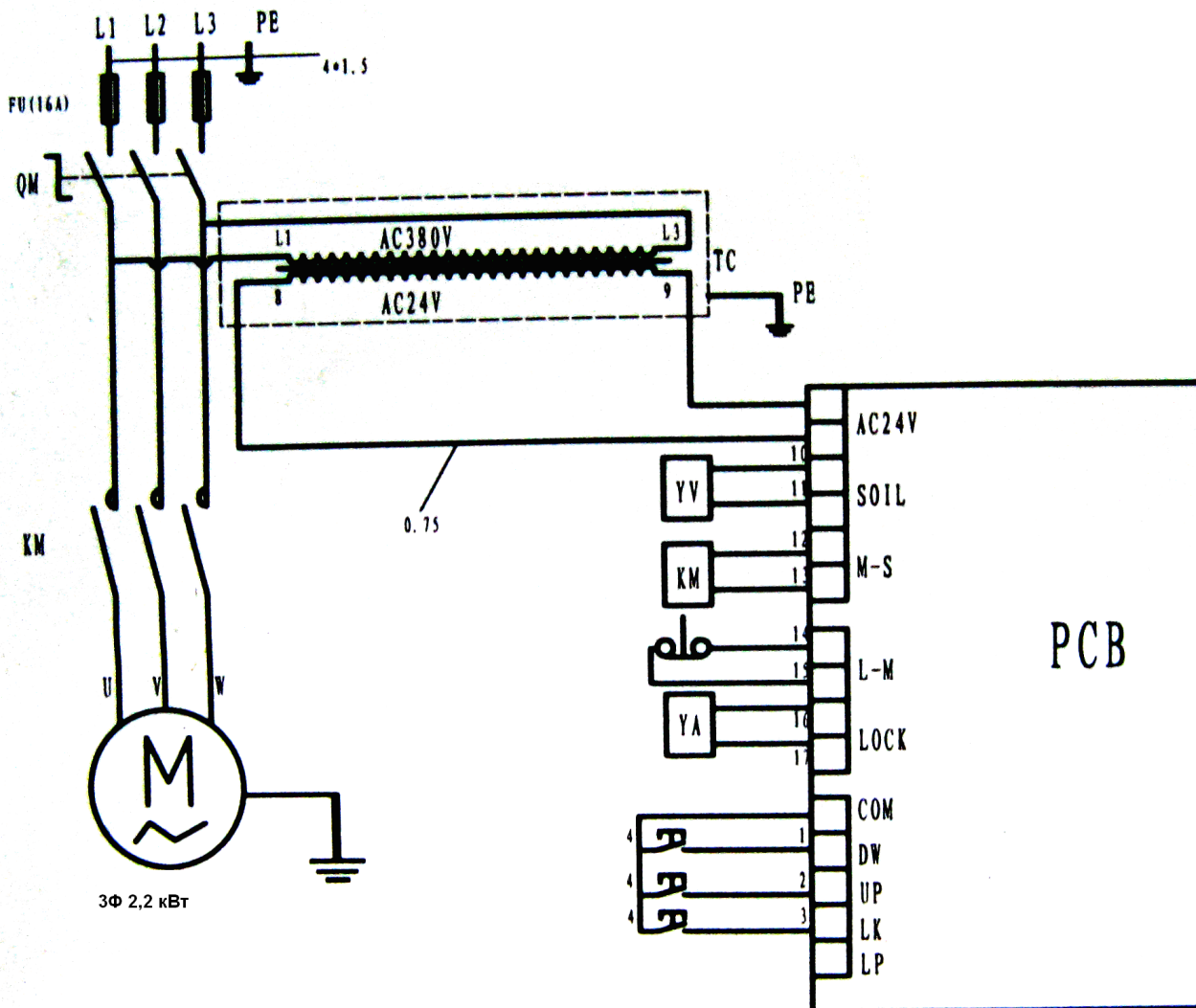
Рис. 5.1 – Электрическая схема
