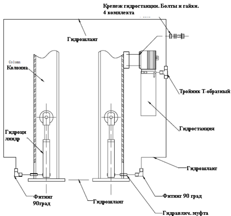
Рис. 4.1 – Гидравлическая схема
