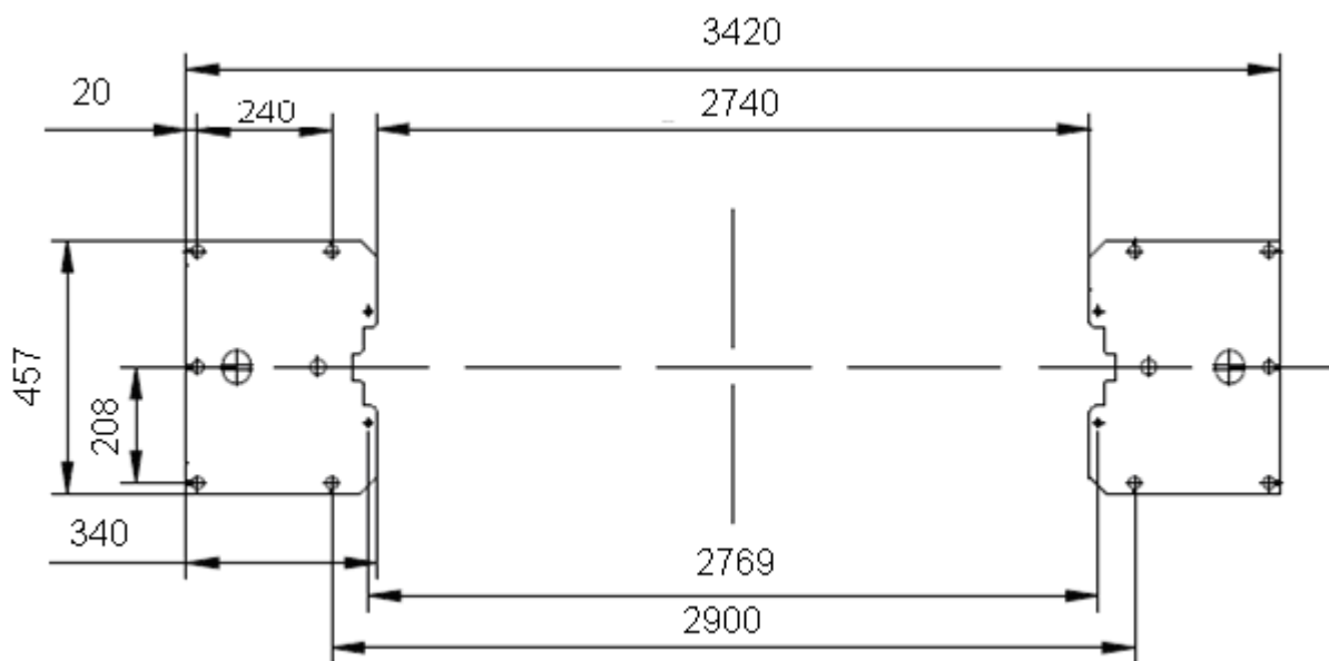
Рис. 3.2 - Установочные размеры
