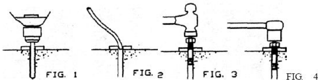
Рис. 2.5 – Установка анкеров
