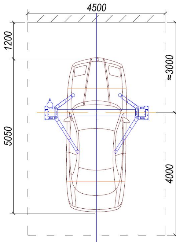
Рис. 1.3 – Рекомендации по размещению автомобиля на подъемнике
