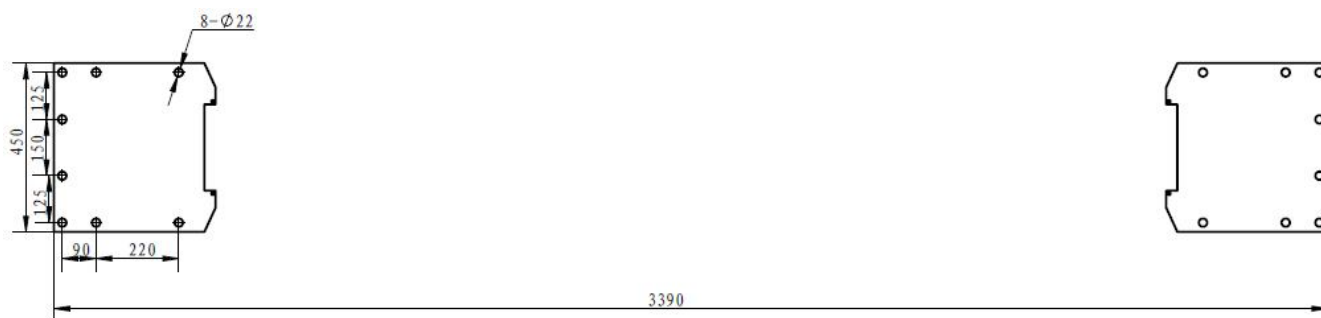
Рис. 3.2 - Установочные размеры
