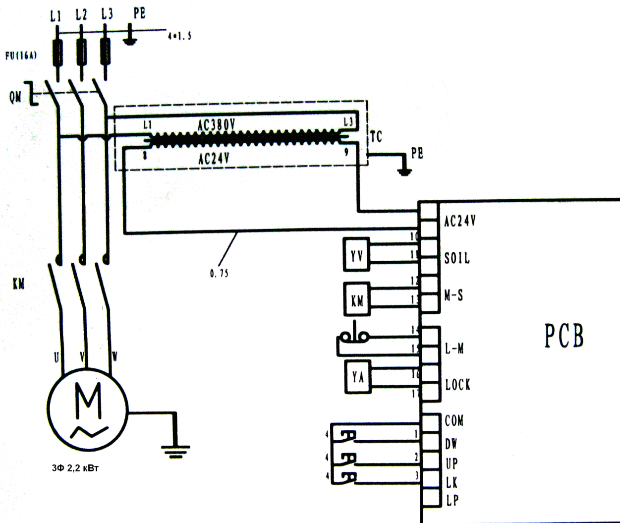
Рис. 5.1 – Электрическая схема
