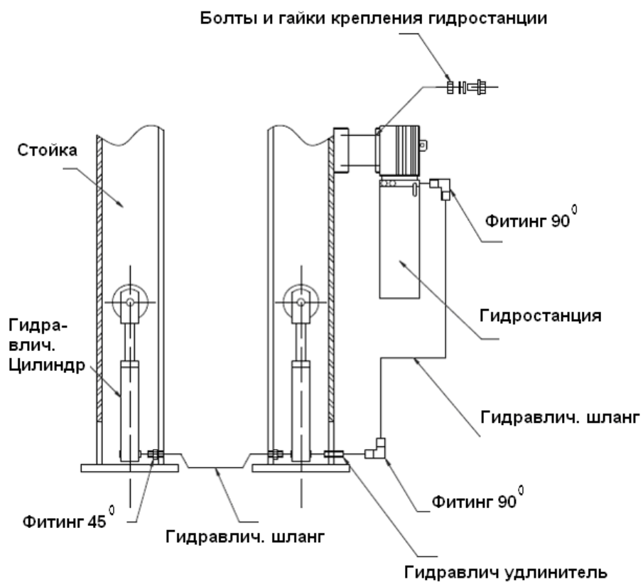
Рис. 4.1 – Гидравлическая схема
