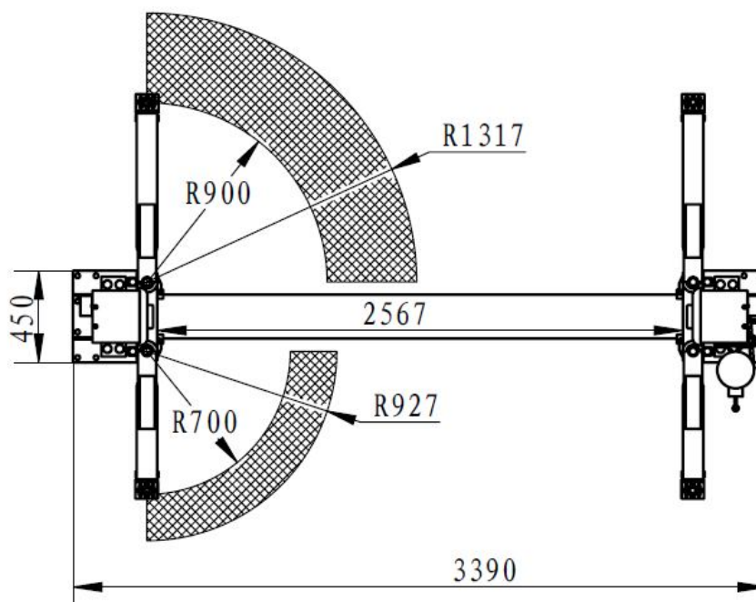
Рис. 1.1 – Габаритные размеры
