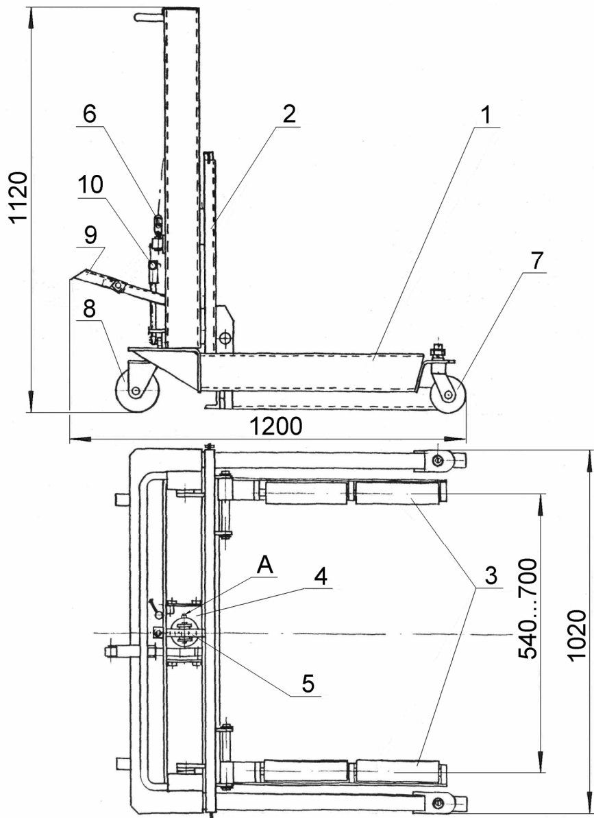
Рис. 1. Тележка ТПП-1
