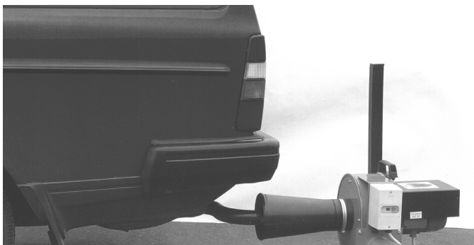
Pict. / Рис. 4 – Правильное расположение установки
