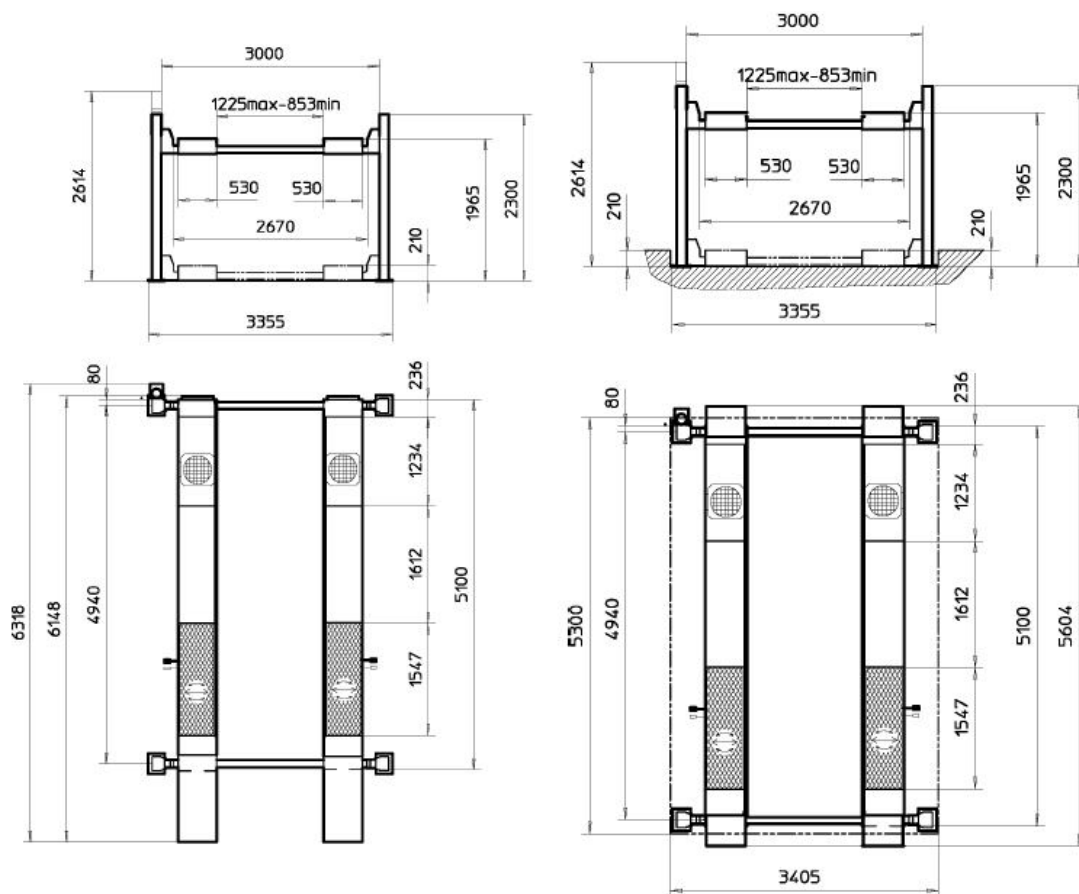
Напольная установка
